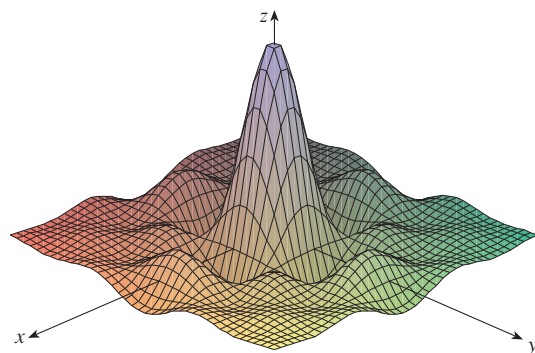
(d) f(x, y) = \frac{\sin x \sin y}{xy}
